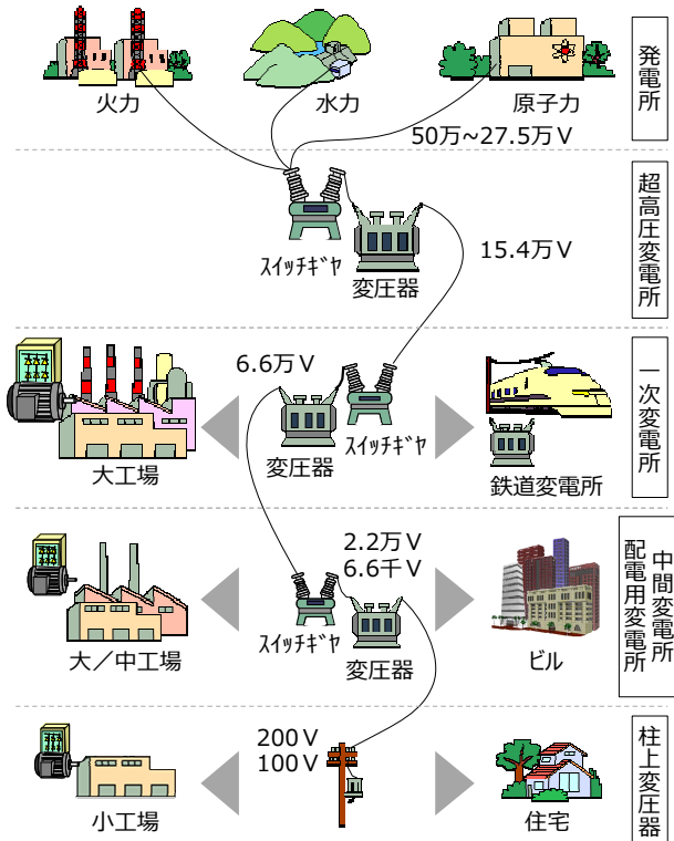
図 1.1 電力供給の経路
